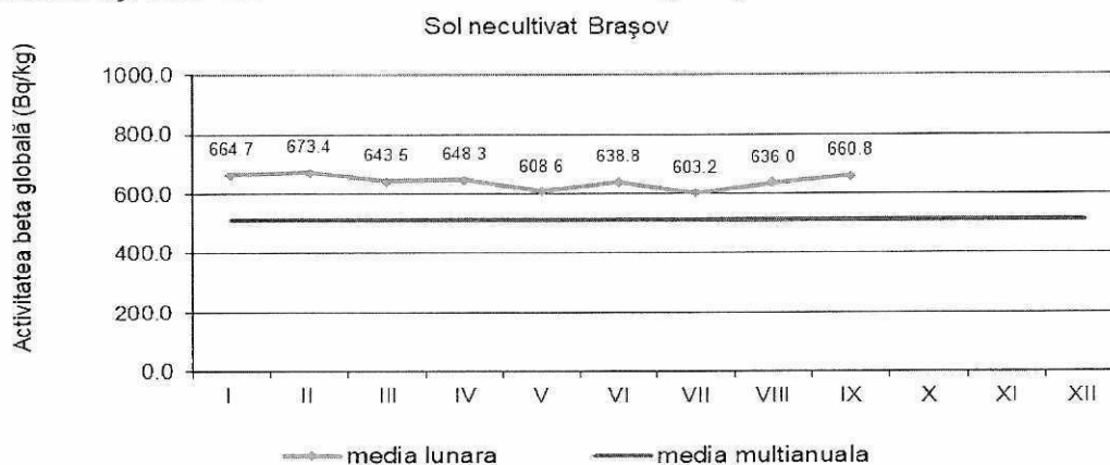
Fig. 1.2.8. Activitatea beta globală la 5 zile pentru solul necultivat
