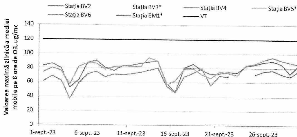
*captura de date valide în luna septembrie a fost de 0% la stația BV3, la stația BV5 și la stația EM1 din motive tehnice Figura 1.1.2.3.2. Evoluția concentrațiilor maximelor zilnice ale mediilor mobile pe 8 ore de O_3 în luna septembrie
