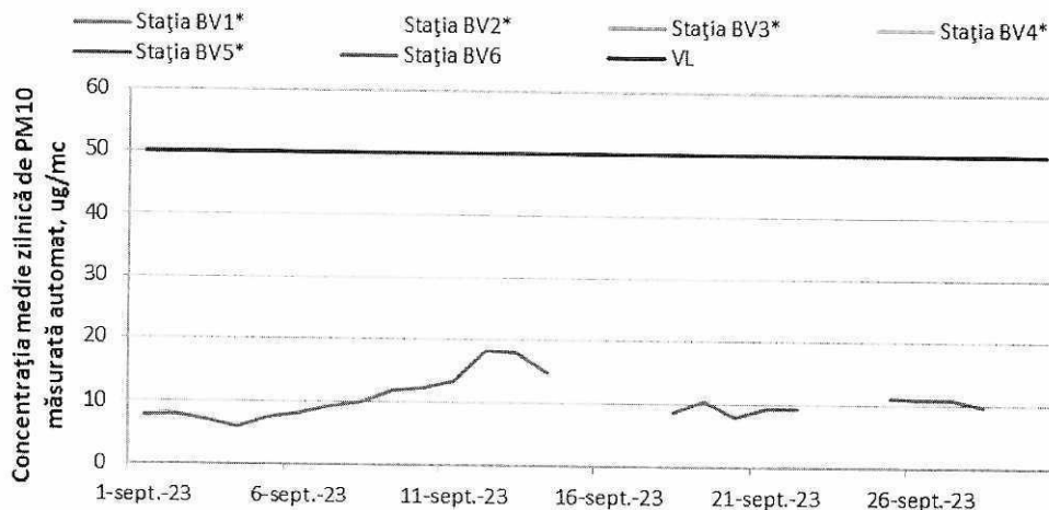
Figura 1.1.2.4.3. Evoluția mediilor zilnice de PM 10, metoda automată, în luna septembrie
