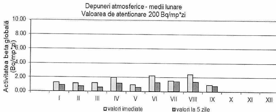
Fig. 1.2.4. Activitatea beta globală pentru depuneri atmosferice
