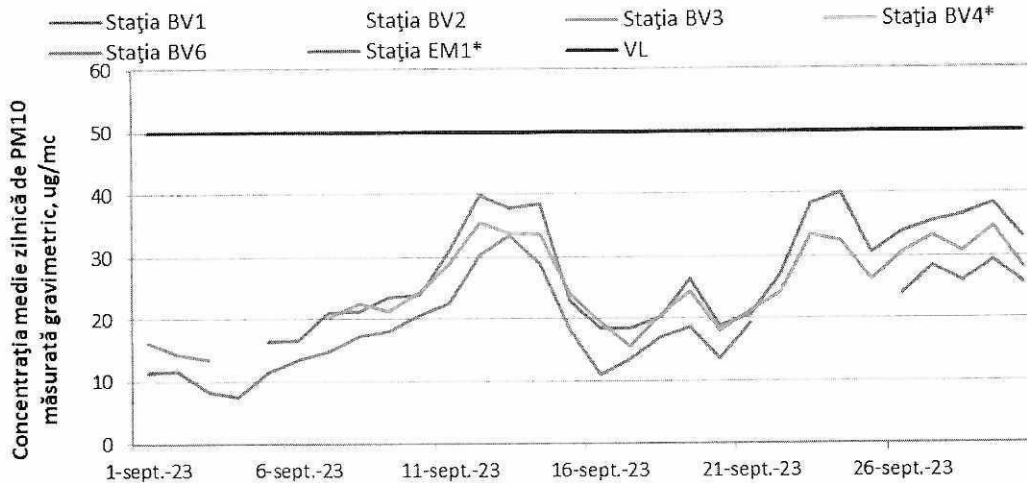
Figura 1.1.2.4.1. Evoluția mediilor zilnice de PM 10 (gravimetric) în luna septembrie
