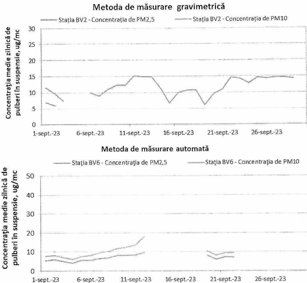
Figura 1.1.2.4.4 Evoluția mediilor zilnice de PM 2,5 și PM10 în luna septembrie
