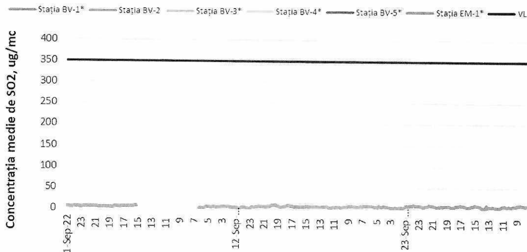
Figura 1.1.2.1.2. Evoluția mediilor orare de SO 2 în luna septembrie
