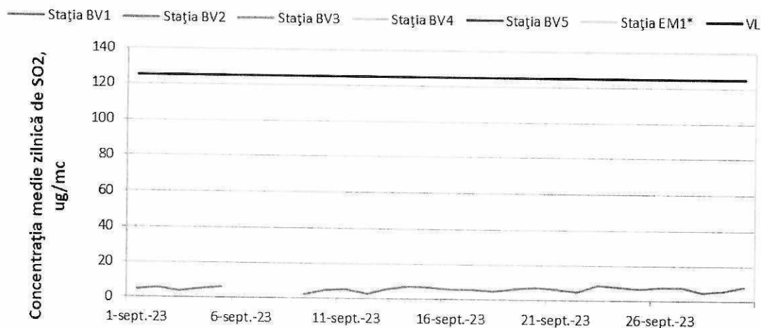
Figura 1.1.2.1.1. Evoluția mediilor zilnice de SO 2 în luna septembrie
